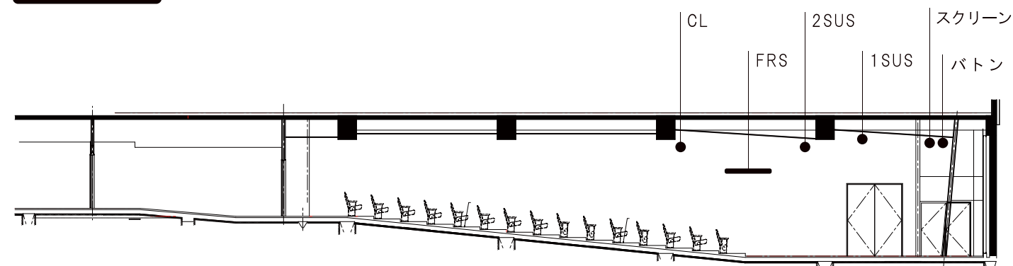
ホール断面図
