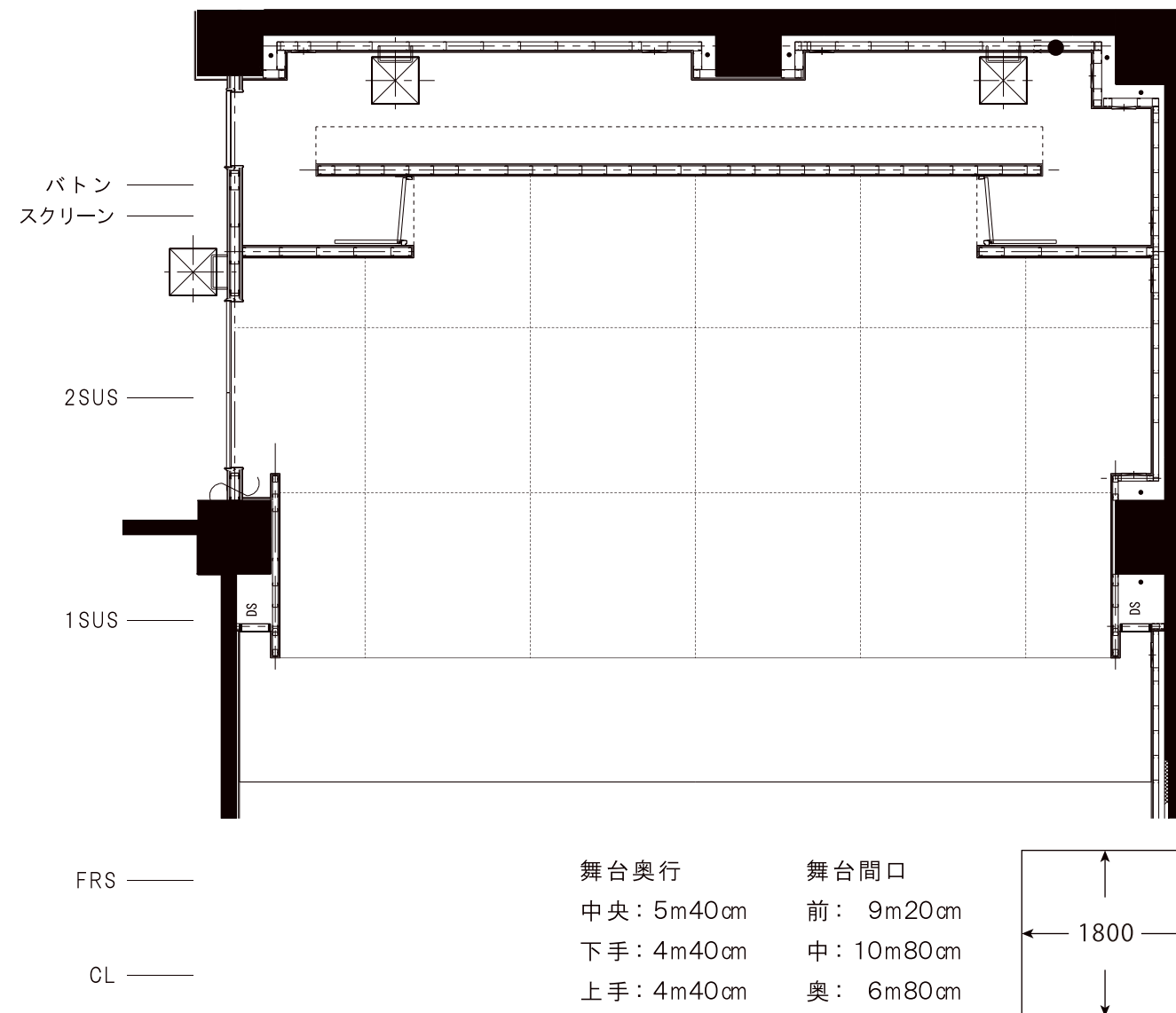
舞台平面図
